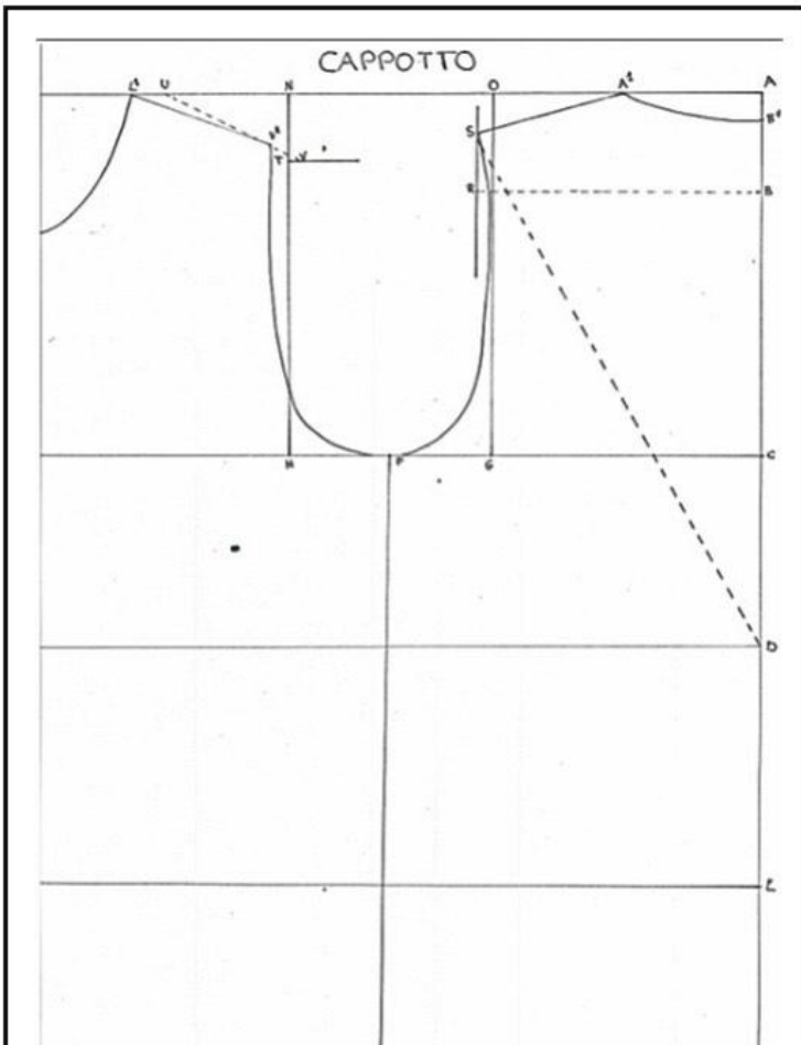
Studio dei capi spalla: Il cappotto base davanti e dietro
